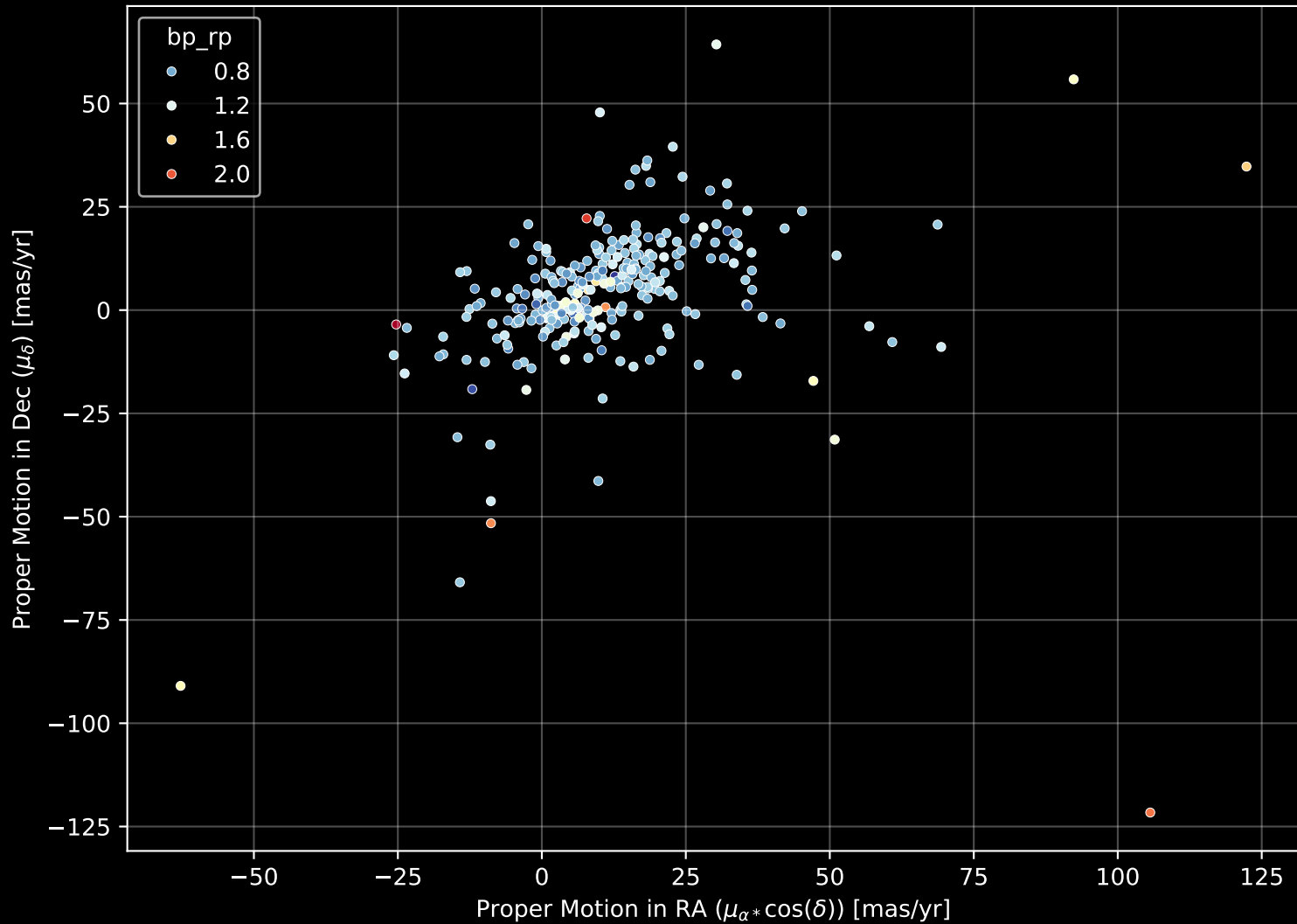
GALAH DR4 Field: [269] Proper Motion Diagram (n= 287)
