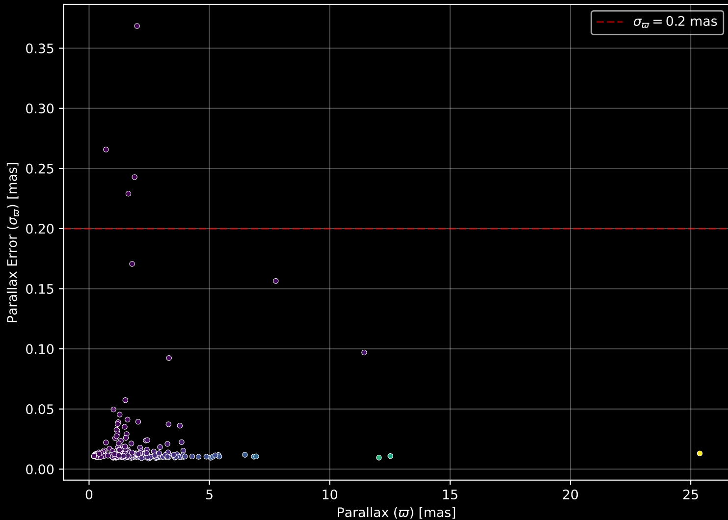
GALAH DR4 Field: [269] Parallax Quality (n= 287)
