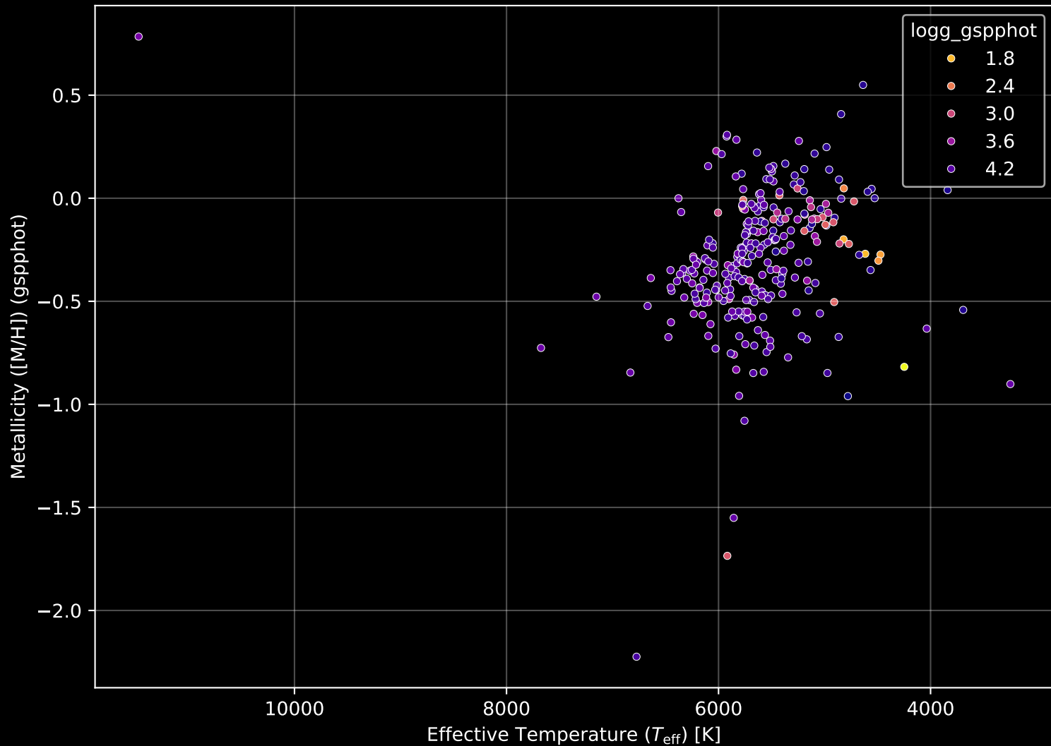
GALAH DR4 Field: [269] Stellar Population Parameters (n= 287)
