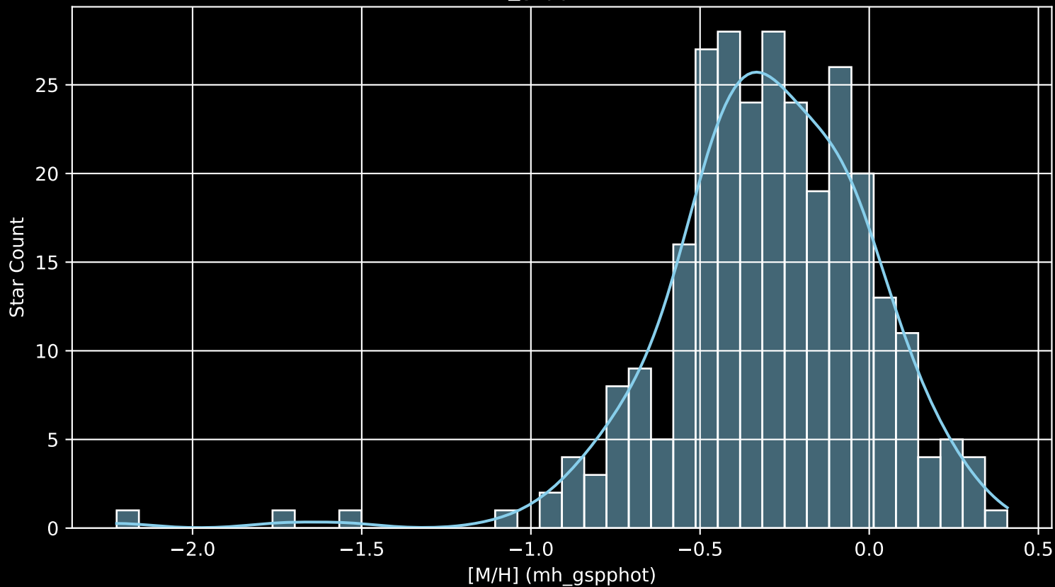
GALAH DR4 Field: [269] [M/H] (mh_gspphot) (n= 285)
